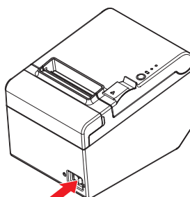
Wasserdichte Netzschalterabdeckung
